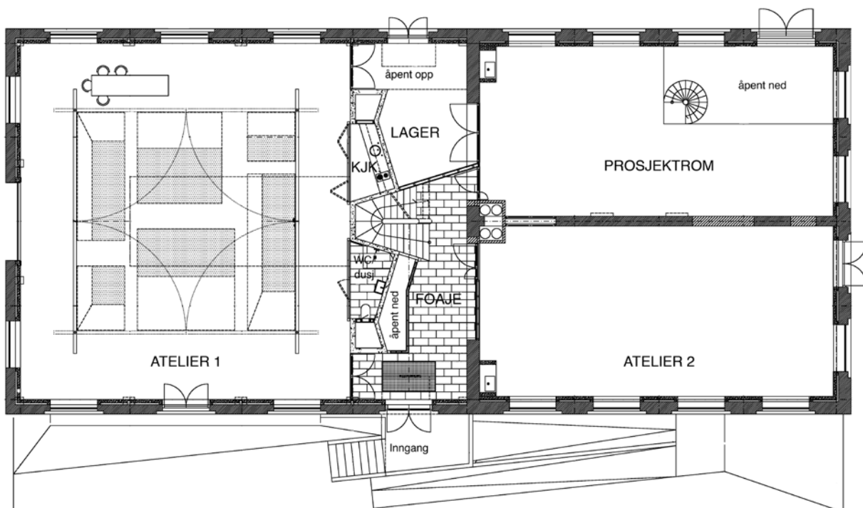
Plan 1. etasje
