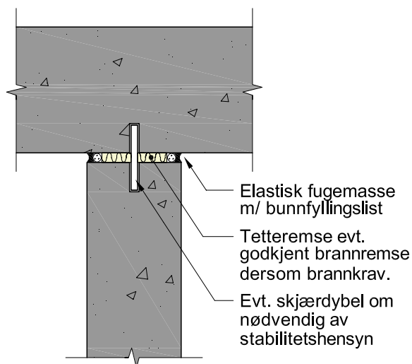
Figur 4: Tetting mot fukt, lyd og evt. brann mellom mur og overliggende dekke.
