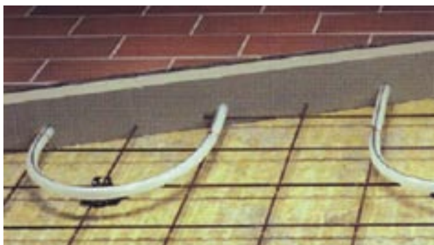
Figur 1: Varmeslyng på armeringsnett
